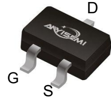
SOT-23-3L
